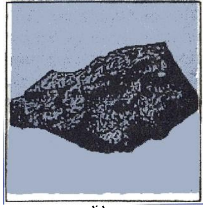
आलेंदे उल्का
